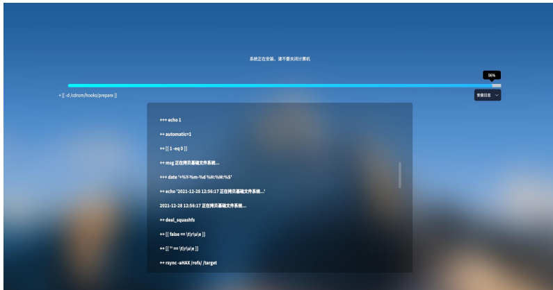
图 11 系统安装日志
