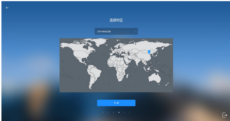
图 5 选择时区
