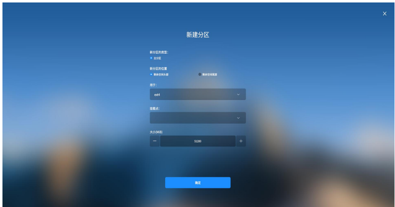
图 15 创建分区
