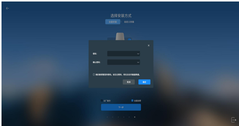
图 8 全盘加密
