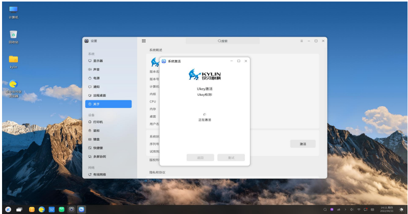
图 28 Ukey 激活
