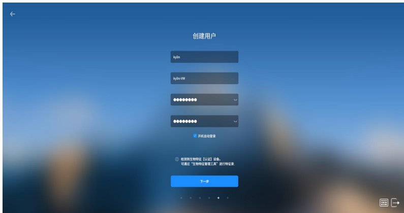
图 6 创建用户
