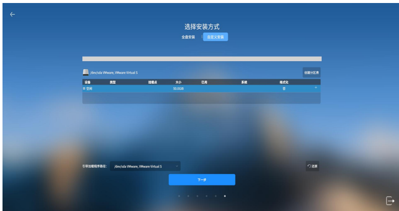
图 14 自定义安装
